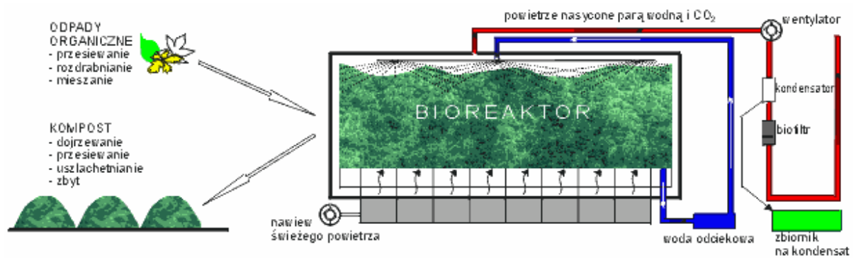
rys. nr 2 - Schemat kompostowni - dla przesegregowanych odpadów
